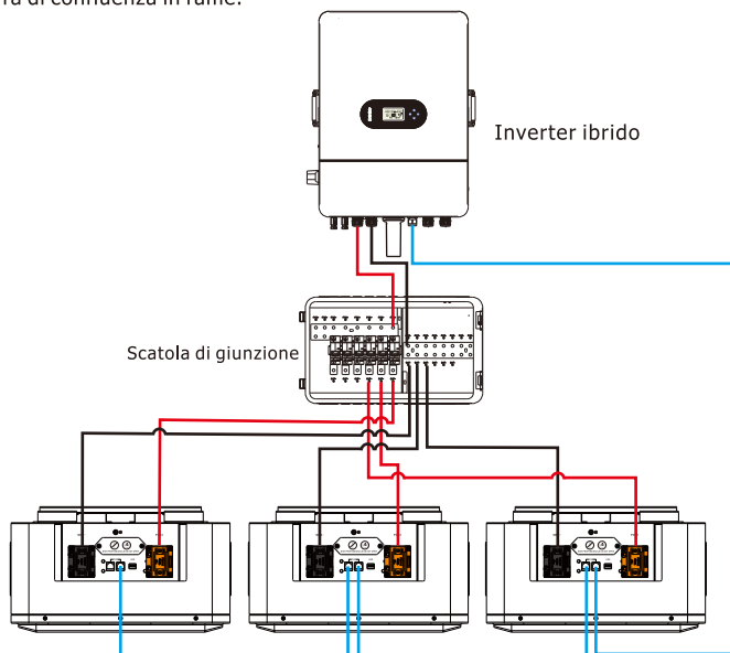
Figura 4-1 Collegamento in parallelo di tre pacchi batteria
