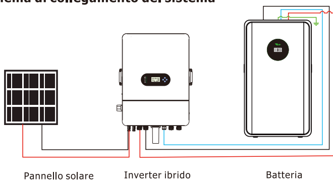
Figura 3-1 Schema di collegamento del sistema a batteria singola
