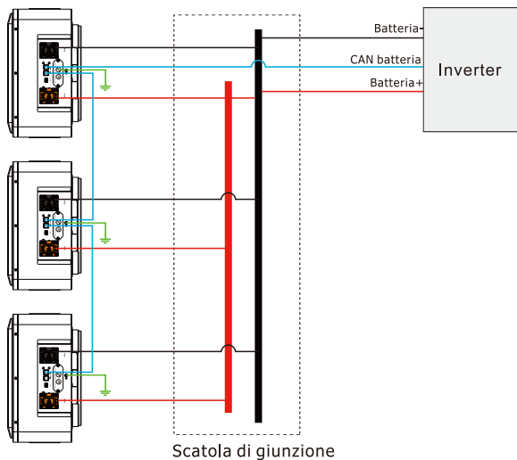
Figura 4-1 Collegamento in parallelo di tre pacchi batteria
