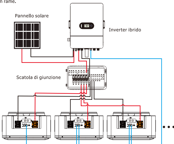
Figura 3-2 Schema di collegamento del sistema a batterie multiple in parallelo
